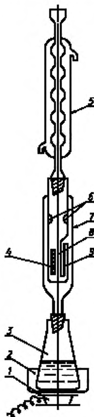
Установка для проведения горячей экстракции полимера
