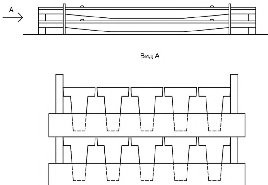
Рисунок 1 — Складирование прогонов
