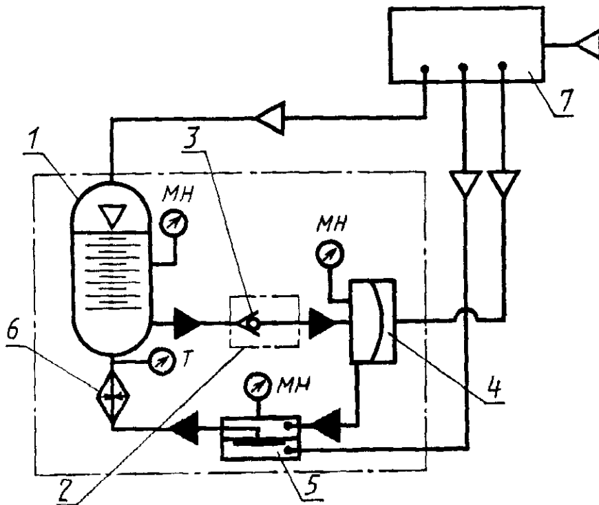
Принципиальная схема стенда для испытания биологических клапанов
