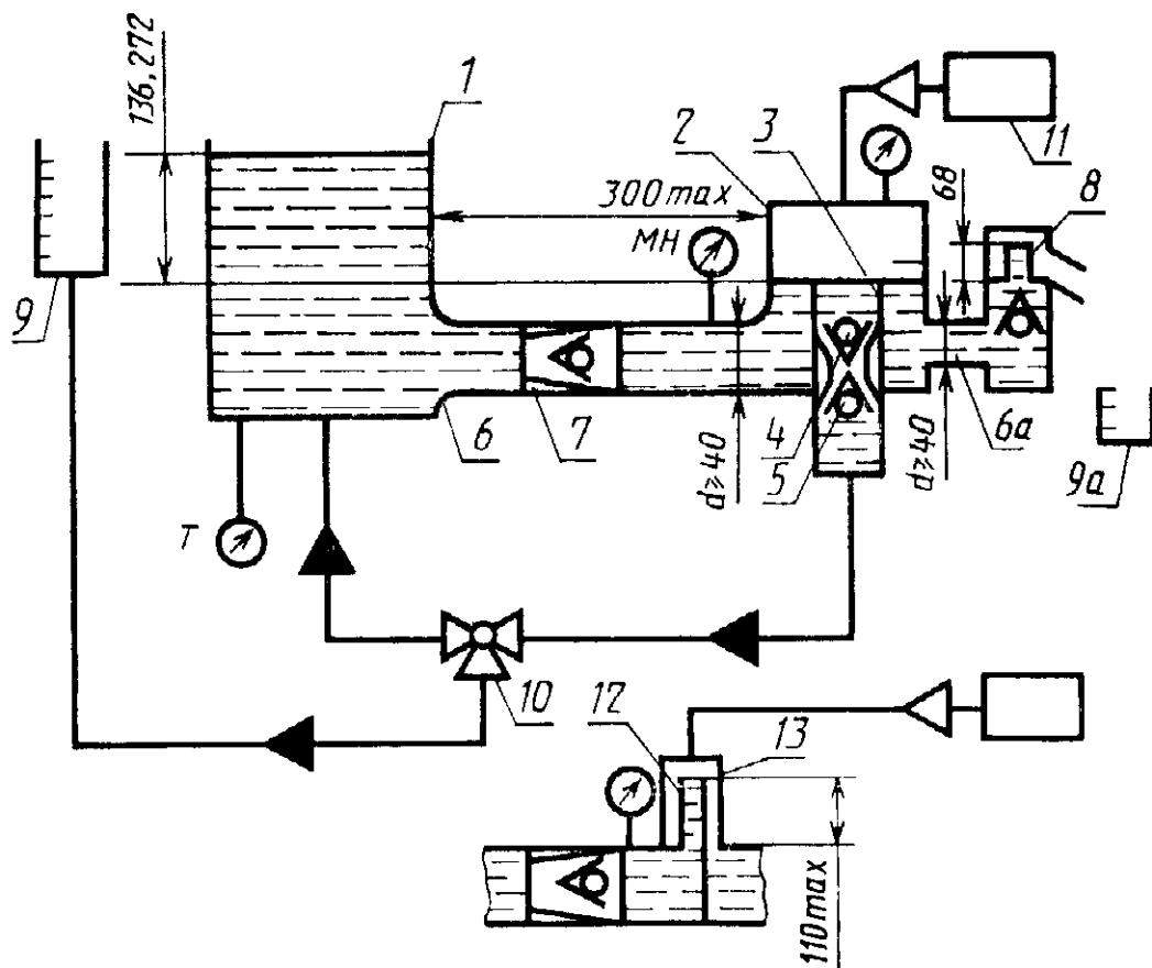
Принципиальная схема стенда для испытания клапанов сердца на пропускную способность и обратный переток
