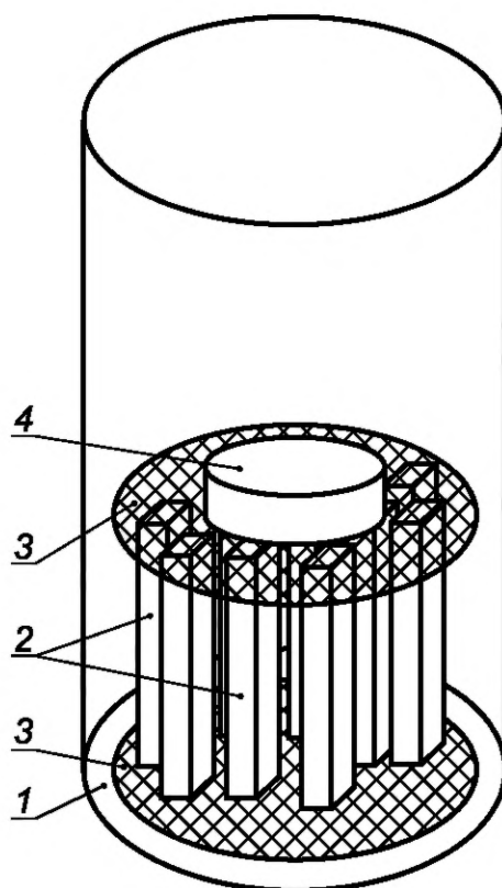
1 — химический стакан; 2 — образцы древесины для испытания; 3 — сетка; 4 — противовсплывное устройство
