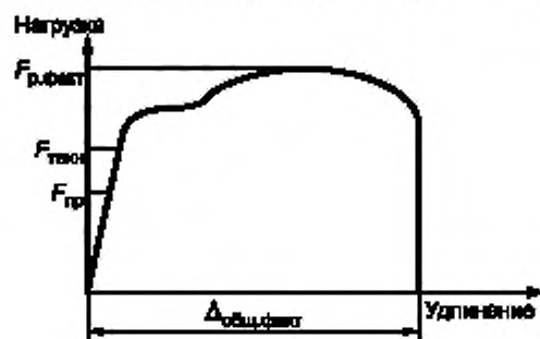
F_{\text{факт}} — фактическая разрушающая нагрузка; F_{\text{техн}} — технологическая нагрузка; F_{\text{пр}} — приемочная пробная нагрузка; \Delta_{\text{общ.факт}} — общее удлинение (фактическое)
