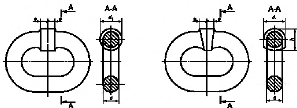
d — калибр; d_1 — диаметр материала, измеренный в месте сварки; h — толщина звена в месте сварки; e — длина сварного шва в каждую сторону от середины звена
