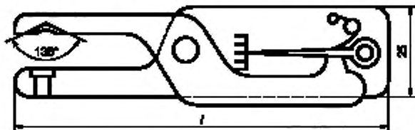
Рисунок В.1 — Шаблон для измерений
