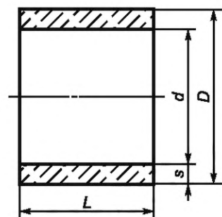
Рисунок 2 — Безнапорная муфта
