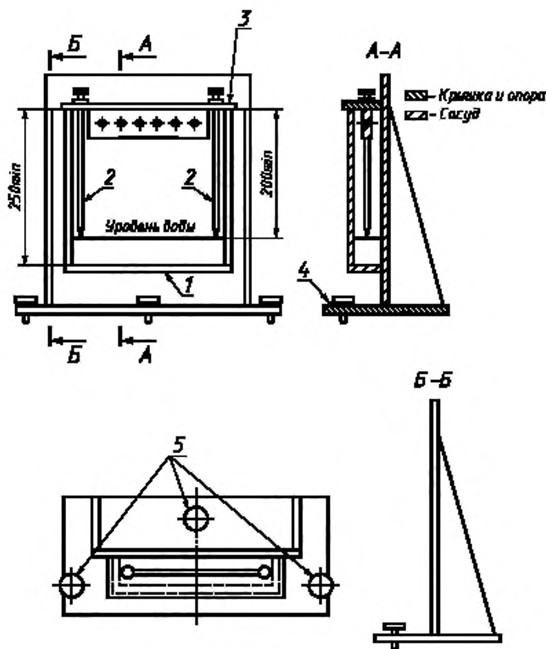
Рисунок 2 — Прибор для определения впитываемости воды
