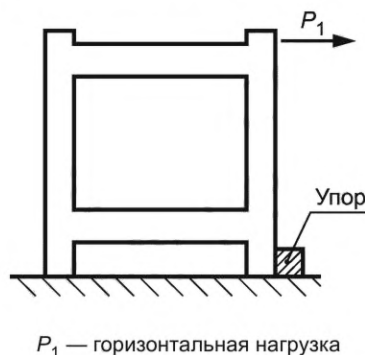
Рисунок 1 — Испытание на устойчивость кровати
