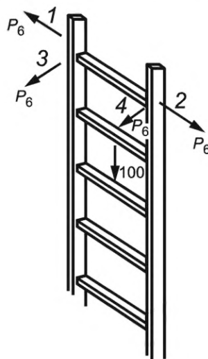
Рисунок 7 — Направление нагружения вертикальных стоек лестницы
