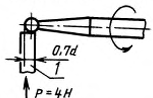
Схема установки боров полостного шаровидного и полостного обратноконусного
