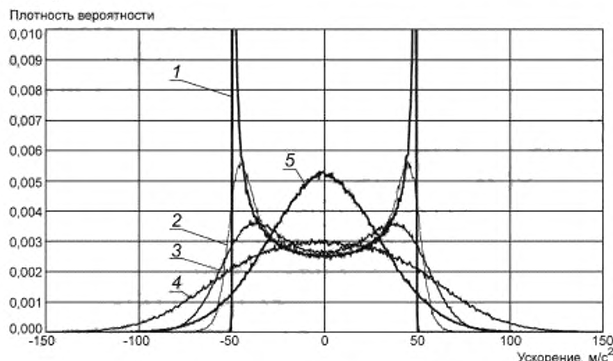
1 — чисто гармонический сигнал; 2 — гармонический и случайный (СПУ — 0,1 \text{ м}^2/\text{с}^3 ) сигналы; 3 — гармонический и случайный (СПУ — 1 \text{ м}^2/\text{с}^3 ) сигналы; 4 — гармонический и случайный (СПУ — 5 \text{ м}^2/\text{с}^3 ) сигналы; 5 — чисто случайный сигнал (СПУ — 5 \text{ м}^2/\text{с}^3 )
