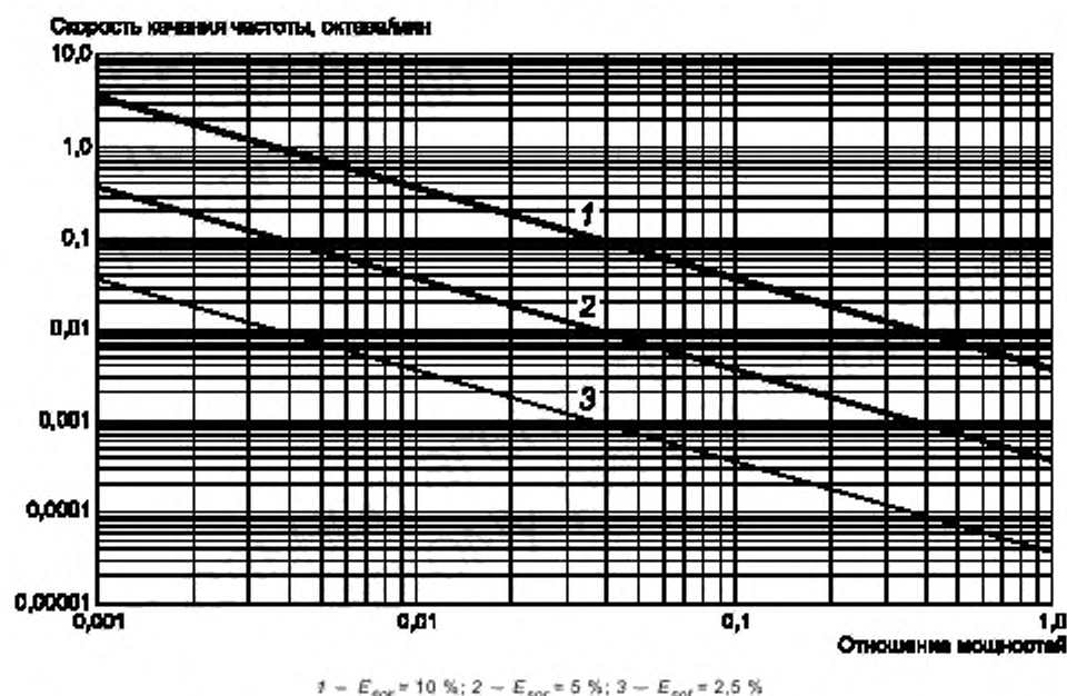
Рисунок 5 — Рекомендуемая скорость качания частоты в зависимости от отношения мощностей для разных значений E_{sot}
