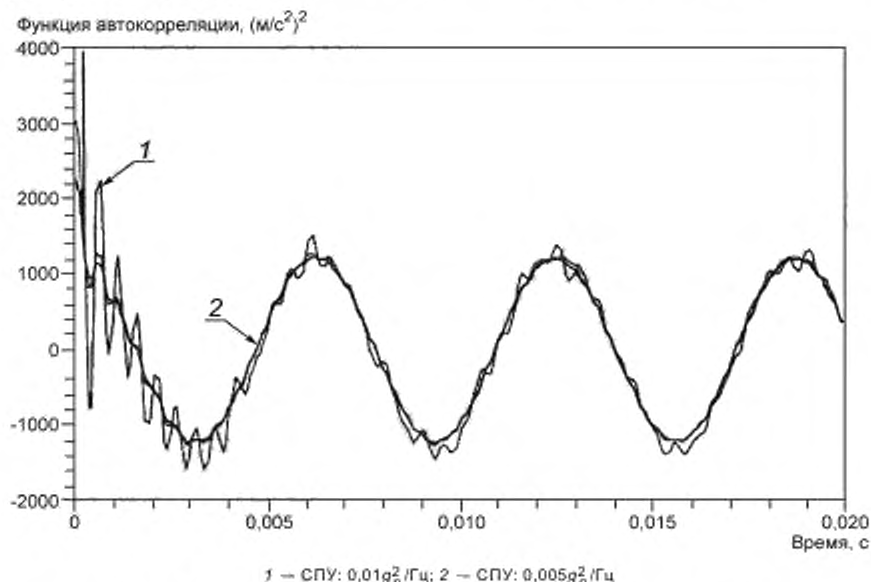
Рисунок А.3 — Автокорреляционная функция для смеси случайного шума с гармоническим сигналом на частоте 160 Гц
