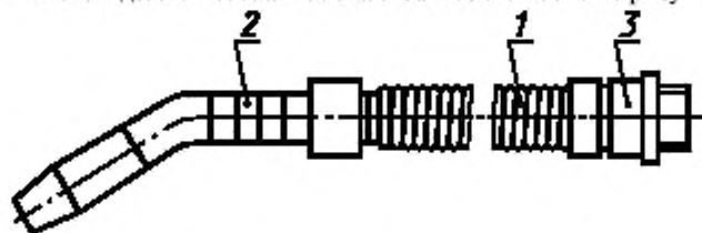
1 — рукав; 2 — наконечник; 3 — патрубок
