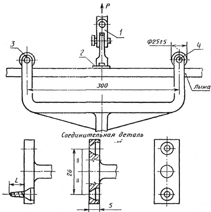
1 — зажимное приспособление испытательной машины; 2 — соединительная деталь; 3 — опора; 4 — свободновращающаяся точка опоры (валек); L — глубина проникания шурупа
