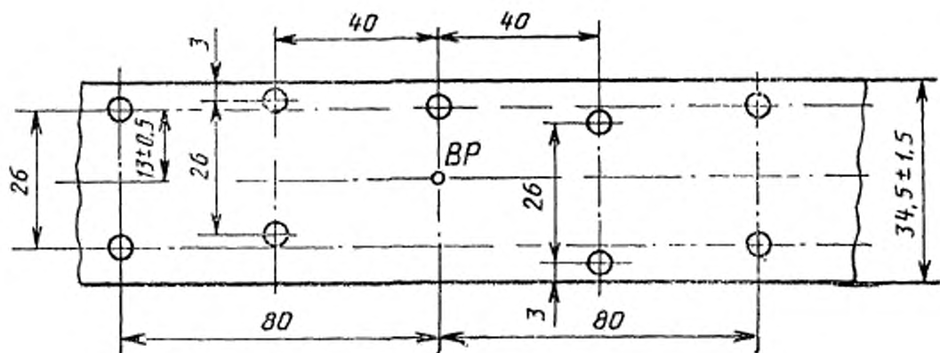
Рисунок 7 — Соединительная деталь
