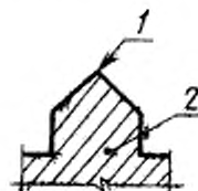
1 — радиус кривизны опоры (макс 0,25 мм); 2 — опора
