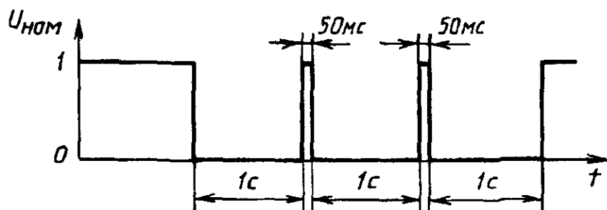
Рисунок 1 — Прерывания напряжения \Delta U=100\% , 1\text{ с}
