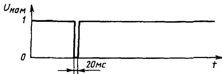
Рисунок 2 — Прерывания напряжения \Delta U=100\% , 20\text{ мс}
