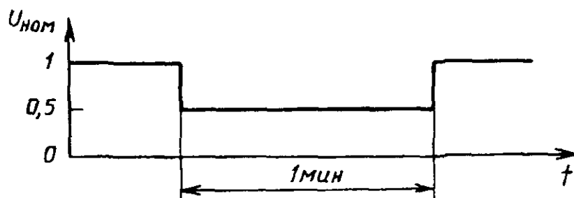
Рисунок 3 — Провалы напряжения \Delta U=50\%
