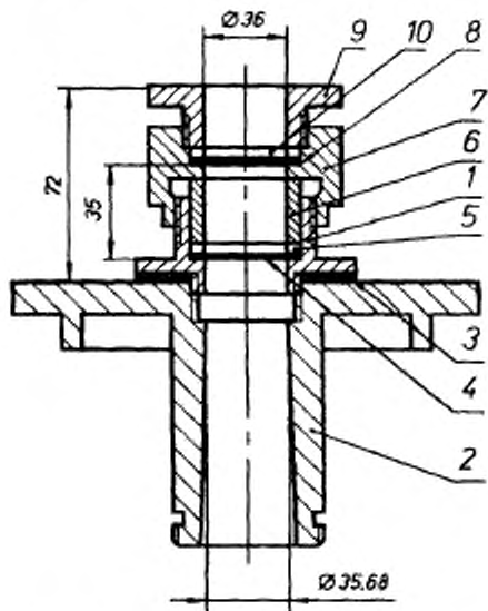
1 — корпус; 2 — сменный столик; 3, 5, 10 — прокладки; 4 — фильтр; 6 — втулка; 7 — гайка; 8 — элементарная проба, 9 — винт
