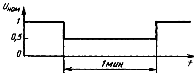
Рисунок 3 — Провалы напряжения \Delta U = 50\%
