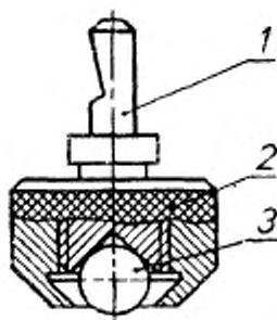
1 — хвостовик наконечника; 2 — гайка наконечника; 3 — шарик
