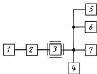
1 — высокочастотный генератор сигнала; 2 — эквивалент антенны приемника; 3 — приемник; 4 — испытательная нагрузка приемника; 5 — низкочастотный частотомер; 6 — низкочастотный вольтметр; 7 — измеритель нелинейных искажений
