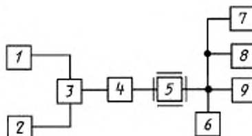
1 и 2 — высокочастотные генераторы сигналов; 3 — согласующее устройство 1-го типа; 4 — эквивалент антенны приемника; 5 — приемник; 6 — испытательная нагрузка приемника; 7 — низкочастотный частотометр; 8 — низкочастотный вольтметр; 9 — измеритель нелинейных искажений
