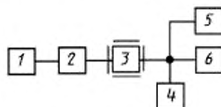
1 — высокочастотный генератор сигнала; 2 — эквивалент антенны приемника; 3 — приемник; 4 — испытательная нагрузка приемника; 5 — низкочастотный частотомер; 6 — низкочастотный вольтметр
