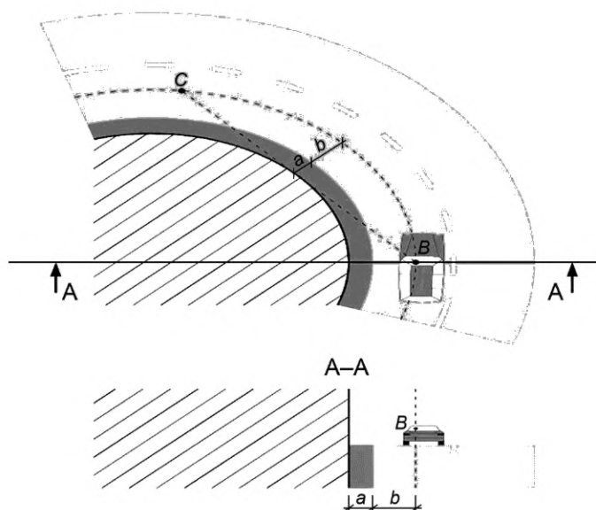
B — положение глаз водителя; C — положение препятствия на проезжей части; b — расстояние от уровня глаз водителя до кромки полосы движения, равное 1,8 м; a — расстояние между кромкой полосы движения и препятствием (шумозащитный экран, барьерное ограждение, откос выемки и др.)
