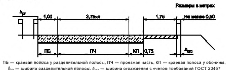
Рисунок 1 — Поперечные профили автомобильных дорог категорий IA, IB, IB с ограждениями
