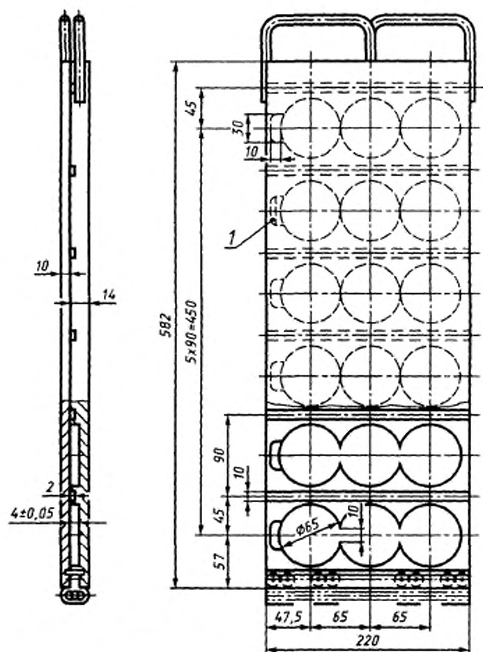
Рисунок 2 — Пресс-форма для вулканизации образцов в виде дисков
