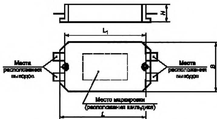
Рисунок А.2 — СЭМ0, вариант исполнения 2
