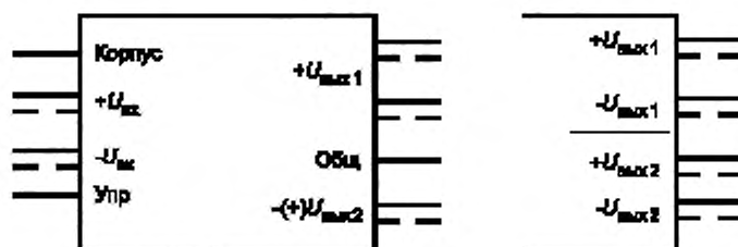
Рисунок Б.2 — Расположение выводов двухканальных СЭМ
