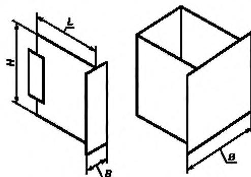
Рисунок 2 — Размеры корпусов СЗМ1
