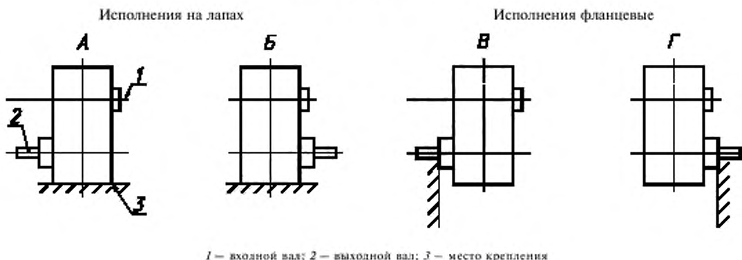
Рисунок А.1 — Варианты сборки
