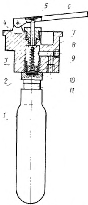
1—баллончик; 2—мембрана; 3—пружина; 4—успокоительное кольцо; 5—шток; 6—рычаг; 7—голова; 8—прижимная втулка; 9, 10—шайба; 11—штуцер баллона
