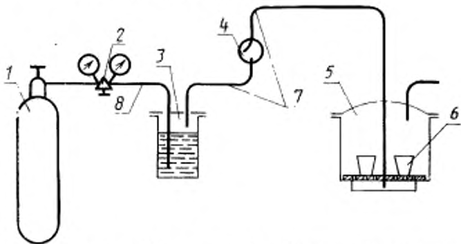
1 - баллон с воздухом; 2 - редуктор газовый; 3 - склянка; 4 - каплеуловитель; 5 - эксикатор; 6 - титал фарфоровые; 7, 8 - трубки соединительные
