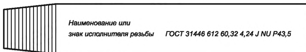
Маркировка краской (рядом с резьбой), нанесенная нарезчиком
