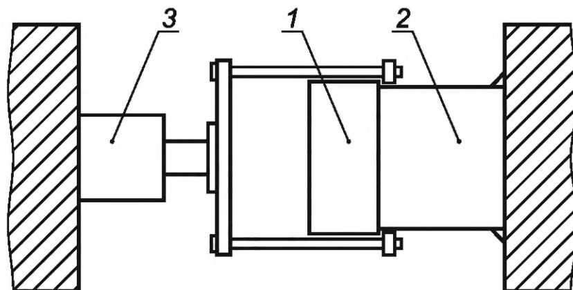
1 — резьбовая предохранительная деталь; 2 — участок трубы; 3 — устройство, для приложения осевой нагрузки
