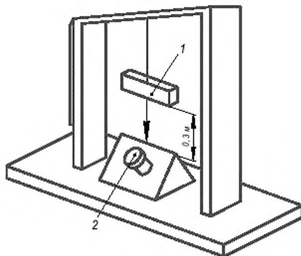
1 – стальная плита; 2 – образец
