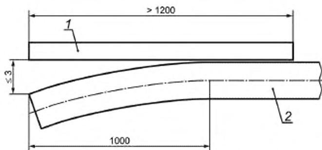
1 — линейка 2 — труба
