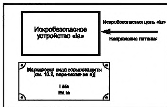
Рисунок 1 — Оборудование уровня взрывозащиты Ma (искробезопасная цепь «ia»)
