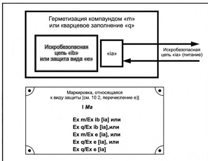
Рисунок 6 — Оборудование уровня взрывозащиты Ma (искробезопасная цепь «ib» или защита вида «е» внутри оболочки с герметизацией компаундом «т» или кварцевым заполнением «q»)
