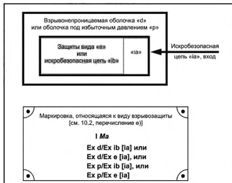
Рисунок 4 — Оборудование уровня взрывозащиты Ma (защита вида «e» или искробезопасная цепь «ib» внутри взрывонепроницаемой оболочки «d» или оболочки под избыточным давлением «p»)
