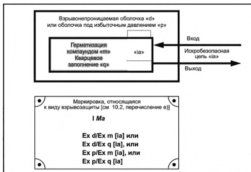
Рисунок 3 — Оборудование уровня взрывозащиты Ma (герметизация компаундом «m» или кварцевое заполнение «q» внутри взрывонепроницаемой оболочки «d» или оболочки под избыточным давлением «p»)
