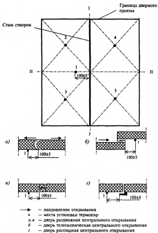
Рисунок А.2 — Схема установки термодатчиков на необогреваемой поверхности двухстворчатой двери
