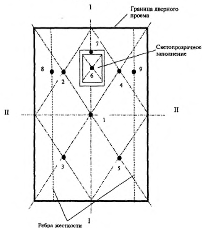
Рисунок А.1 — Схема установки термопар на необогреваемой поверхности створок одностворчатой распашной и горизонтально-раздвижной двери бокового открывания с частичным остеклением
