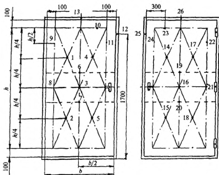
Рисунок 1 — Схема установки термоэлектрических преобразователей (термопар) на необогреваемой поверхности однопольных дверей
