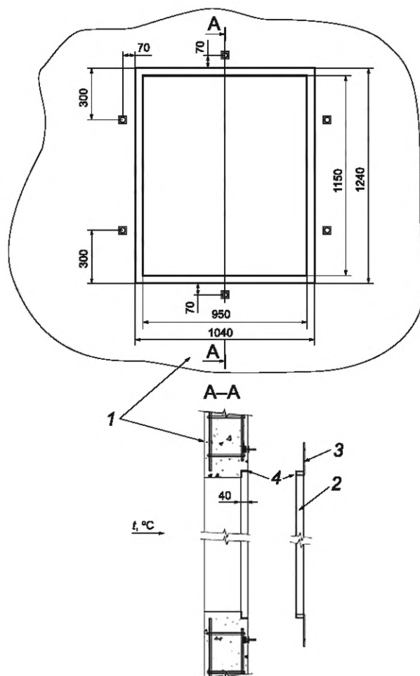
1 — ограждающая конструкция; 2 — монтажное приспособление (рама (40 \times 20 \times 2) \pm 2 мм); 3 — планка крепления; 4 — волокнистый теплоизоляционный материал
