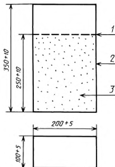
Рисунок А.2 — Мешок с сухим песком
