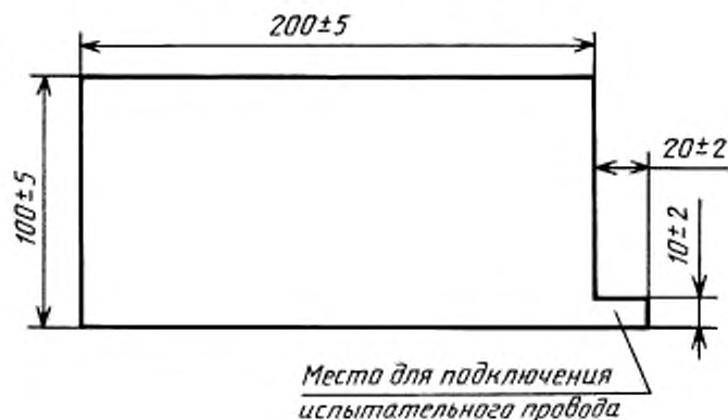
Рисунок А.1 — Электрод из медной фольги
