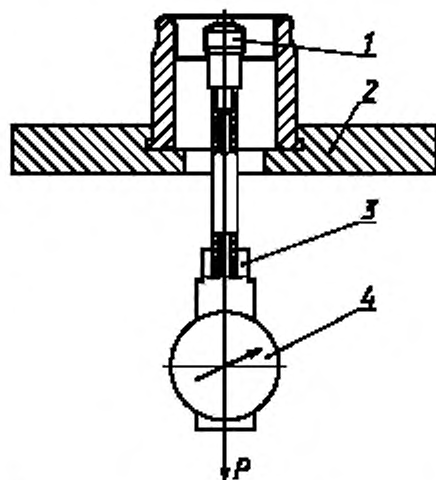
1 — клапан аэрозольный; 2 — основание приспособления; 3 — зажим трубки; 4 — динамометр; Р — прикладываемая сила
