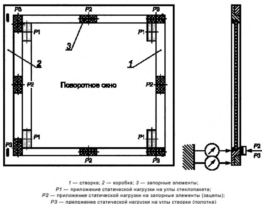
Рисунок Е.1 — Точки приложения статических нагрузок
