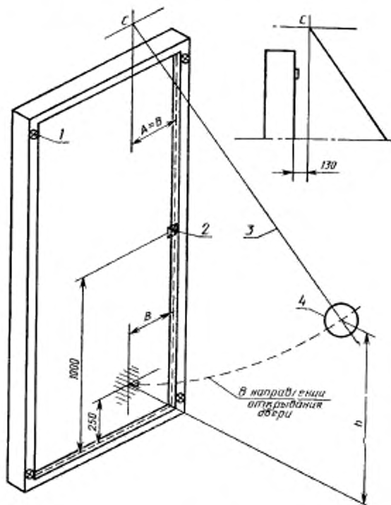
1 — прижим; 2 — запирающий прибор или ограничитель; 3 — гибкая нить; 4 — неупругое тело (груз). B = \frac{1}{2} ширины полотна, но не более 300 мм.
