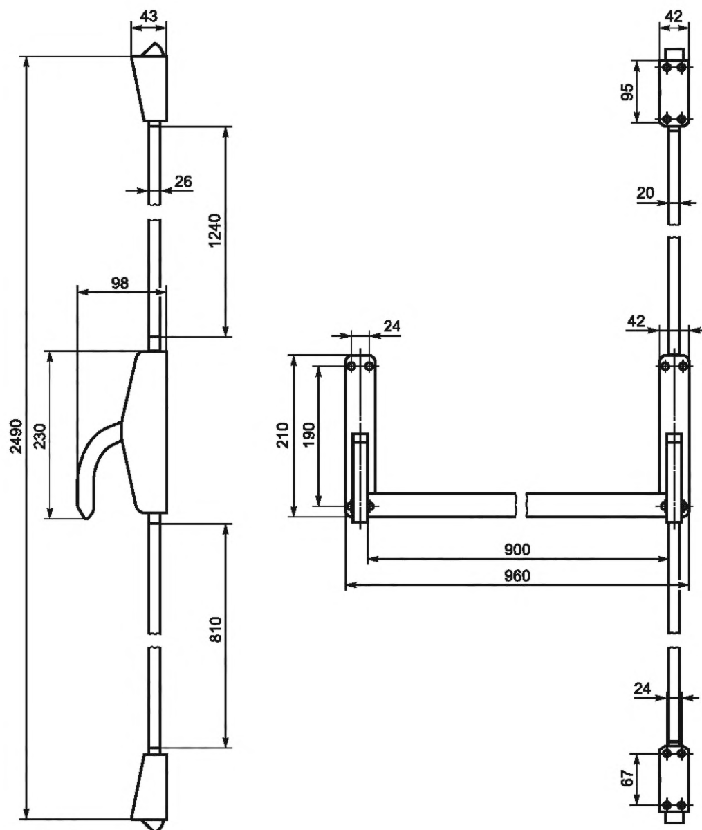
Рисунок А.3 — Пример устройства «Антипаника», управляемого штангой, с запираемостью дверей эвакуационных выходов в трех точках
