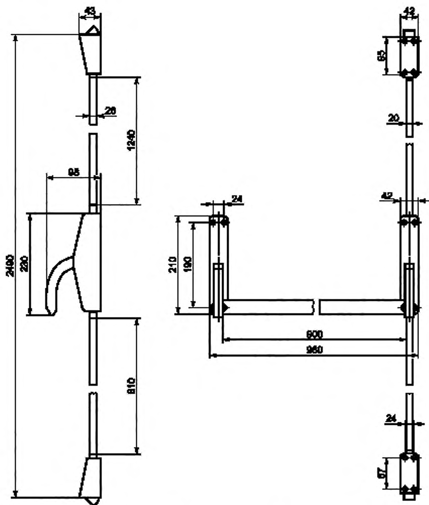
Рисунок А.3 – Пример устройства «Антипаника», управляемого штангой, с запирающим дверей эвакуационных выходов в трех точках
