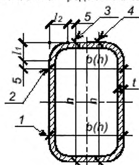
Рисунок 3 – Схема измерения размеров квадратных и прямоугольных профилей
