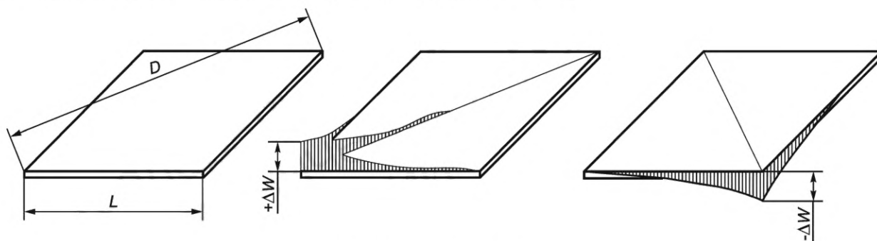
Рисунок 6 — Коробление
