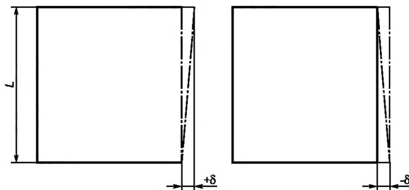
Рисунок 3 — Косоугольность
