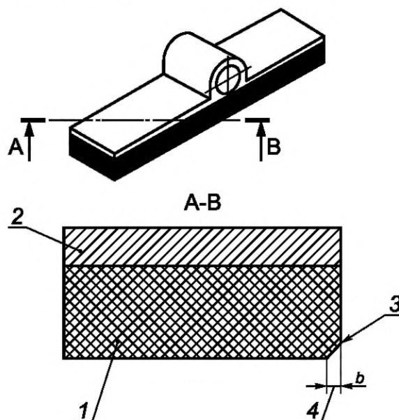
Рисунок 26 — Ползун, демонстрирующий максимальный износ на ударной кромке
