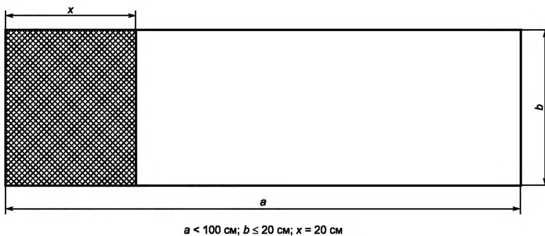
Рисунок 9 — Схема выборки образцов из прямоугольной плитки с площадью лицевой поверхности 400 - 3600 \text{ см}^2
