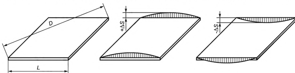
Рисунок 5 — Выпуклость/вогнутость граней
