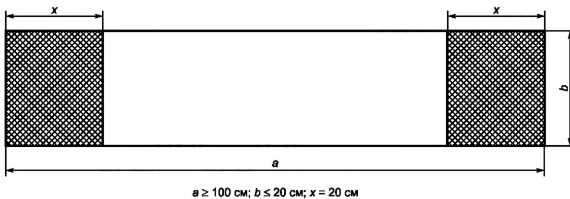
Рисунок 10 — Схема выборки образцов из прямоугольной плитки с площадью лицевой поверхности \geq 400 \text{ см}^2
