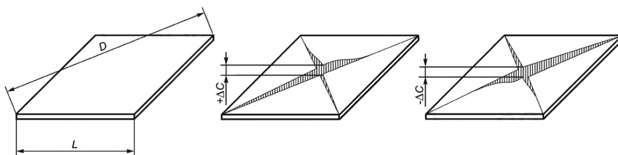
Рисунок 4 — Выпуклость/вогнутость по центру
