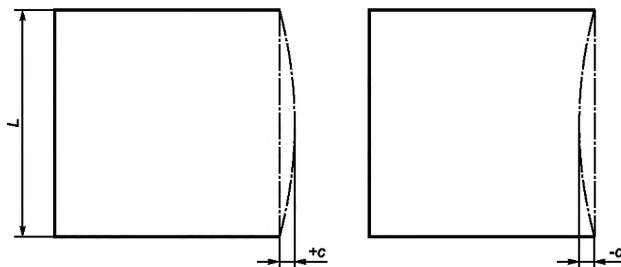
Рисунок 1 — Прямолинейность граней
