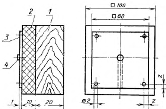
1—деталь из твердой древесины; 2—термоизоляционный материал, коэффициент теплопроводности которого при 30°C 0,04—0,047 Вт/(м·К); 3—медная пластина; 4—термодатчик
