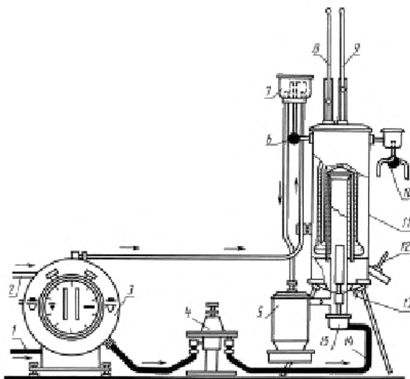
1 — газопровод; 2 — водопровод; 3 — газовый счетчик; 4 — мембранный регулятор давления высокой чувствительности; 5 — увлажнитель воздуха; 6 — вентиль для регулирования воды; 7 — переливной бак для воды; 8, 9 — термометр для измерения температуры воды на выходе; 10 — трехходовый кран для нагретой воды; 11 — теплообменник; 12 — термометр для измерения температуры отходящих газов; 13 — выпускной патрубок конденсата; 14 — шланг газовой горелки; 15 — газовая горелка
