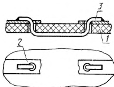
1 — материал основания; 2 — поврежденный печатный проводник; 3 — перемычка
