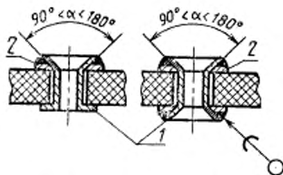
1 — арматура перехода; 2 — контактная площадка
