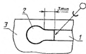
1 — печатный проводник; 2 — новая контактная площадка; 3 — материал основания
