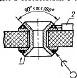
1 — арматура перехода; 2 — перемычка
