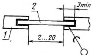
1 — поврежденный печатный проводник; 2 — перемычка
