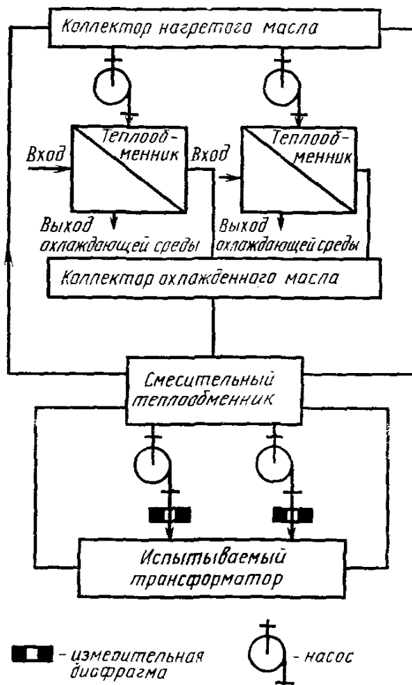
Принципиальная схема установки для испытаний трансформаторов с охлаждением видов Ц и ДЦ без собственной системы охлаждения
