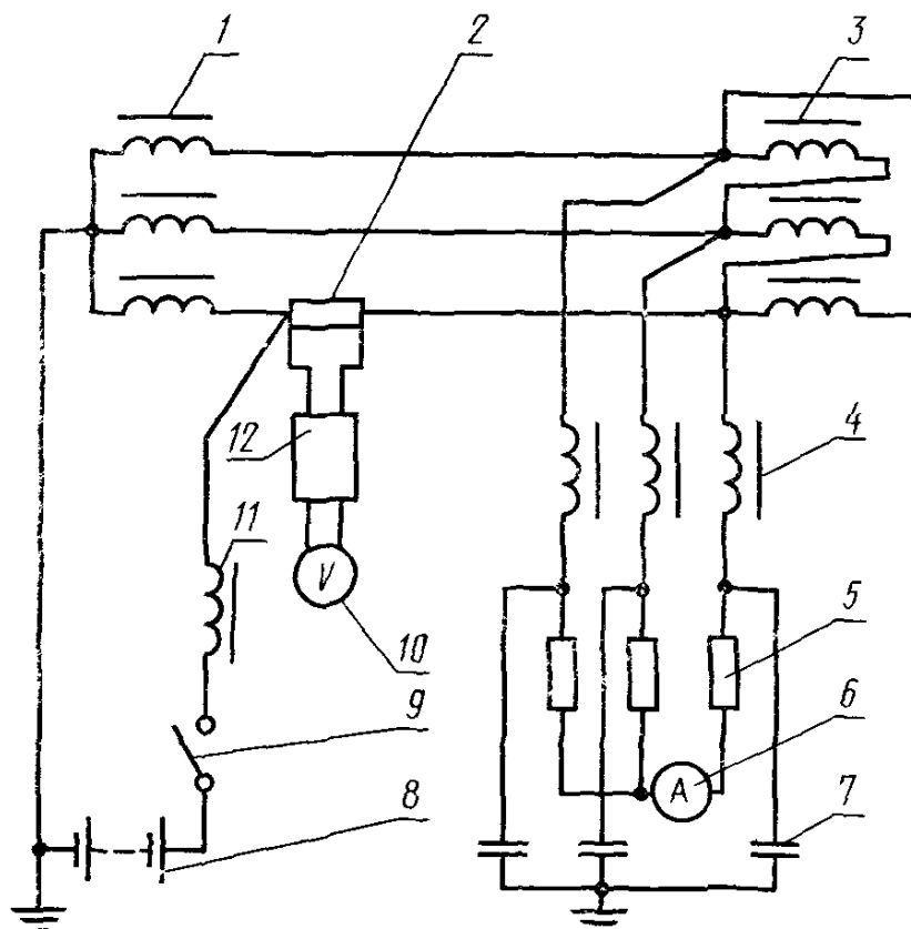
1—питающий трансформатор; 2—шунт; 3—измеряемая обмотка; 4—индуктивность; 5—резистор; 6—микроамперметр; 7—конденсатор; 8—аккумуляторная батарея; 9—выключатель; 10—милли- вольтметр; 11—дрессель; 12—фильтр
