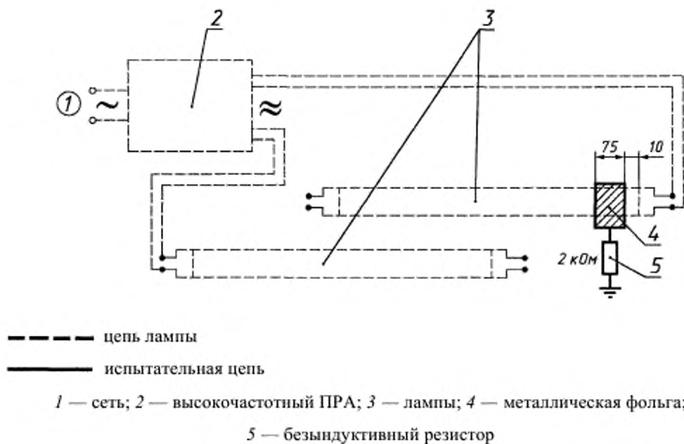
Рисунок 4 — Испытательное устройство
