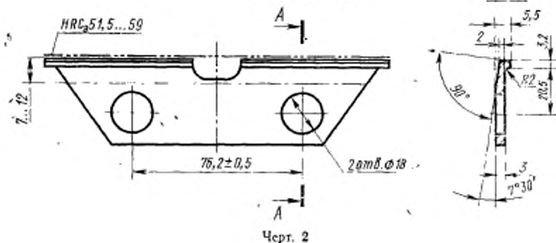
Тип 1 Исполнение 2
