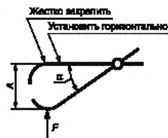
A — размер, установленный конкретно для каждого типа инструмента, \alpha = 25^\circ - 45^\circ
