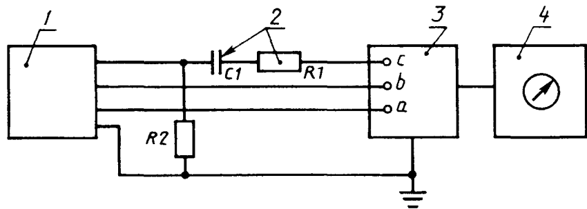
1 — блок питания; 2 — элементы эквивалентной схемы, заменяющей ограждение; 3 — эквивалент сети, 4 — измеритель радиопомех; a, b — сетевые зажимы, c — зажим подключения блока питания, R1 = 250\text{ Ом} , R2 = 1\text{ МОм} (20 кВ); C1 = 10\text{ нФ}
