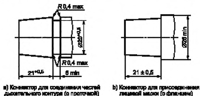
Рисунок 2 — Конические металлические коннекторы размером 22 мм (дополнительные размеры)
