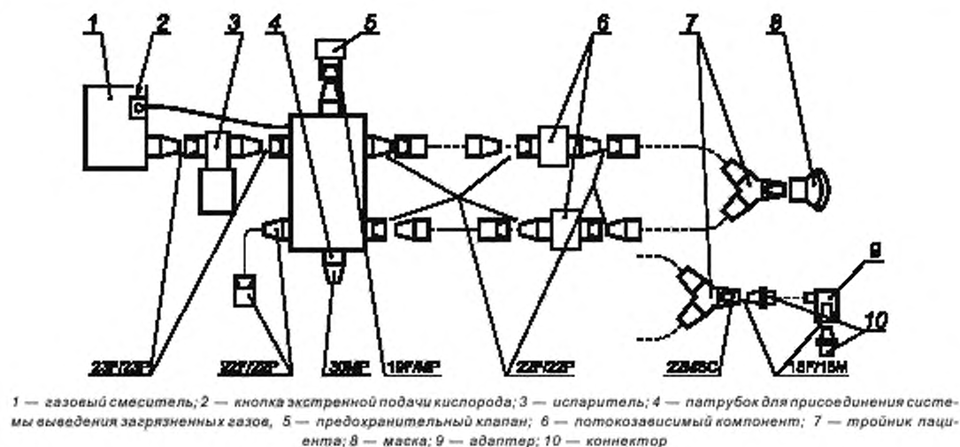
Рисунок Г.2 — Пример применения конических соединений
