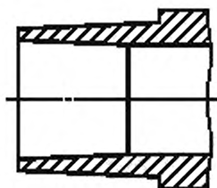
Рисунок Г.1 — Коаксиальная конструкция отверстия для присоединения пациента
