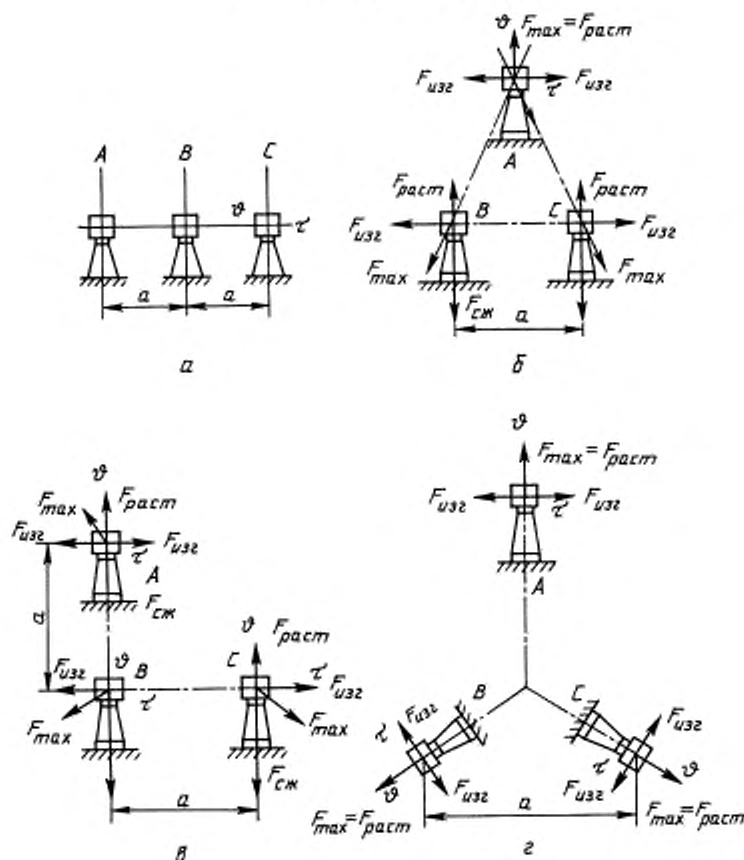
Схемы взаимного расположения шин
