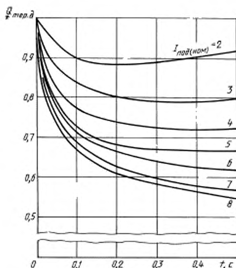
Кривые для определения Q_{\text{тер.д}} от синхронного электродвигателя
