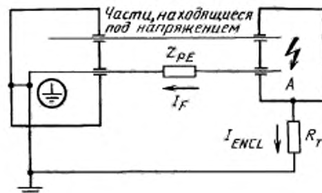
Части ИЗДЕЛИЯ Части, НАХОДЯЩИЕСЯ ПОД НАПРЯЖЕНИЕМ
