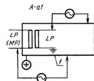
1 — ДОСТУПНАЯ МЕТАЛЛИЧЕСКАЯ ЧАСТЬ
