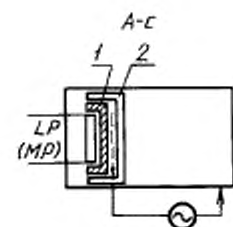
1 — ОСНОВНАЯ ИЗОЛЯЦИЯ; 2 — ДОПОЛНИТЕЛЬНАЯ ИЗОЛЯЦИЯ
