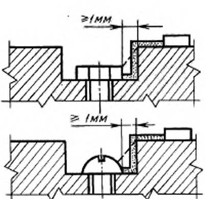
Рисунок 46 — Пример 8 (см. пункт 57.10)
