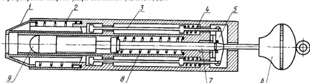
Ударное испытательное устройство (см. раздел 21):
