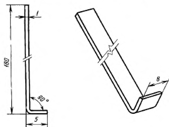
Испытательный крюк (см. раздел 16)
