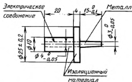
Испытательный штырь (см. раздел 16)
