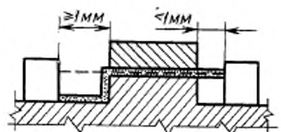
Рисунок 45 — Пример 7 (см. пункт 54.10)
